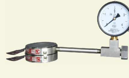
爆破片和安全阀组合 Bursting disc and safety valves combination 使用介质: 气体、液体 Medium: Gas, liquid Std.:ASME VIII-API 526 Sizes: 1"-12" Press.: 0.1MPa ~ 42.0MPa Temp.: 150°C ~ 538°C
