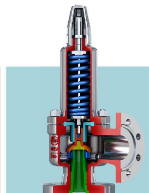
HFA42系列弹簧全启式安全阀 HFA42 Series spring fall lift safety valve 使用介质: 气体、液体 Medium: Gas, liquid Std.:GB/T 12243 Sizes: DN25~400 Press.: PN16 ~ 100 Temp.: -196°C ~ 300°C
