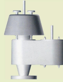
HFHX系列呼吸阀 HFHX Series breather valve 使用介质: 气体 Medium: Gas Std.:ASME VIII-API 526 Press.: Class 150Lb Temp.: ≤200°C
