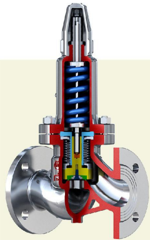
HFAHN42F系列平行式波纹管安全回流阀 HFAHN42F Series balanced bellows safety backflow valve 使用介质: 气体、液体 Medium: Gas, liquid Std.:ASME VIII-API 526 Sizes: 1 1/2"-4" Press.: Class 150Lb ~ 300Lb Temp.: -196°C ~ 200°C
