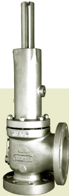
HFB系列弹簧式安全泄压阀 HFB Series spring safety relief valve 使用介质: 气体、液体 Medium: Gas, liquid Std.:ASME VIII-API 526 Sizes: 3/4"-16" Press.: Class 150Lb ~ 2500Lb Temp.: -196°C ~ 300°C
